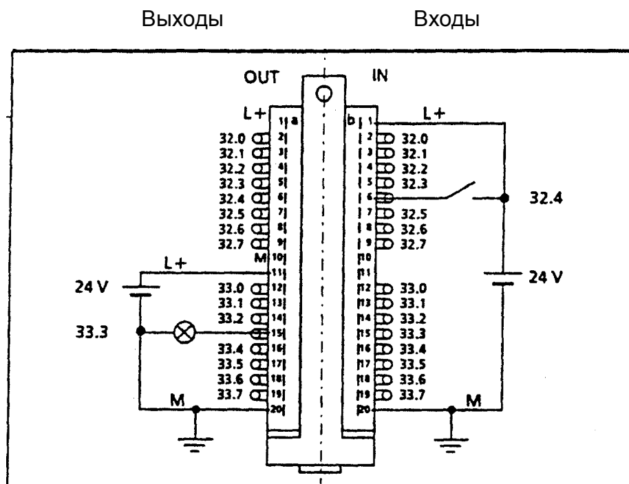
Фигура 1-2 Общий вид переднего разъема цифрового ввода/вывода
